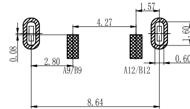
PCB板参考图
